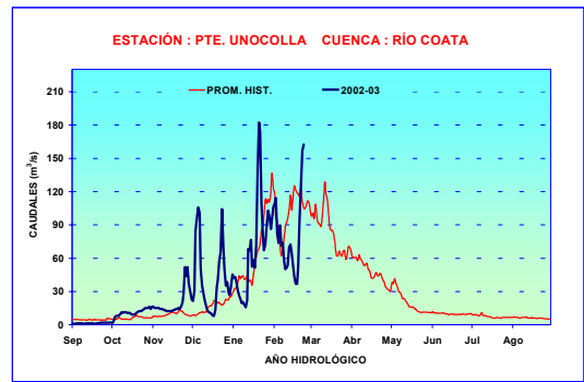
Figura 17. Hidrograma de caudal medio diario del río Coata
