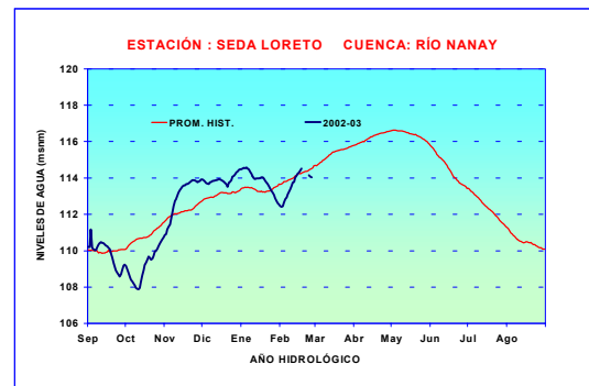
Gráfico 23. Limnigrama de niveles diarios del río Nanay
